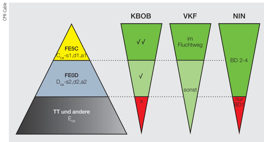
Bild 2 Die Kabel für die unterschiedlichen in der Schweiz geforderten Brandsicherheitsniveaus und ihre Eignung nach den verschiedenen Vorschriften.
