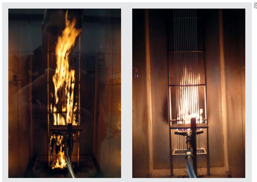
Bild 3 Brandtest, wie er für die beschriebene Klassifizierung (Reaction to Fire) verwendet wird. Links ein Kabel mit niedrigem Sicherheitsniveau, rechts eines mit hohem Sicherheitsniveau.
